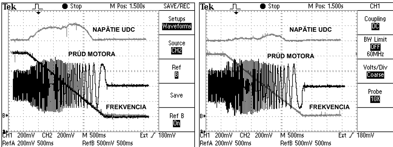
Brzdenie tokom pri menšom zosilnení.
